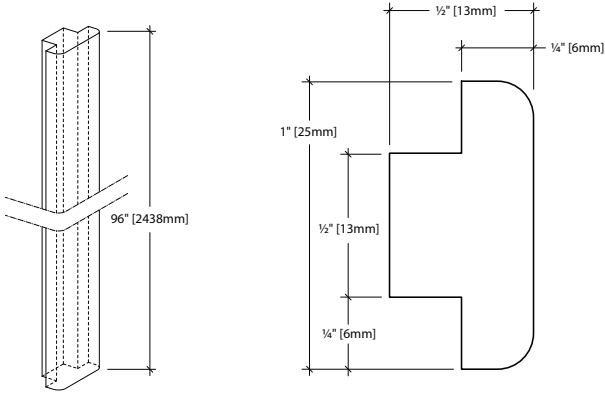
AXONOMETRIC
