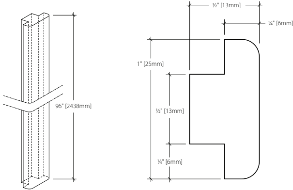
AXONOMETRIC
