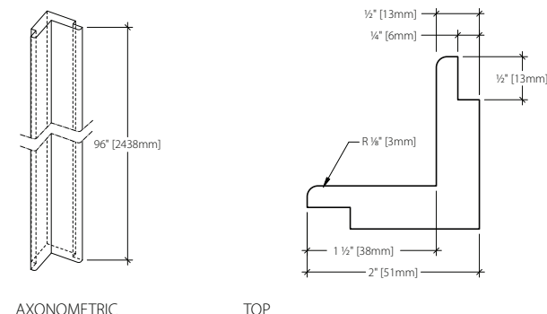
AXONOMETRIC
