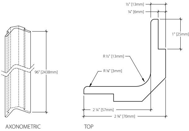
AXONOMETRIC
